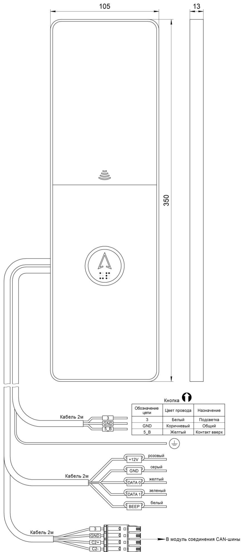
Рис.1 Внешний вид, габаритные и установочные размеры Вызывного поста МАЛАХИТ НШЕК.468381.015-09
